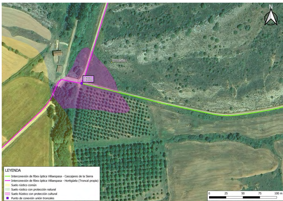
Figura 2. Plano emplazamiento salida Villaespasa.
